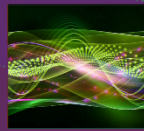
艺术家对超弦的想法。图片来源自维基百科。
