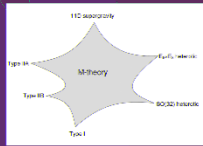
不同的超弦理论通过对偶联系起来。图片来源自维基百科。
