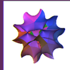
Quintic卡比-丘成桐流的二维截面。图片来源自维基百科。
